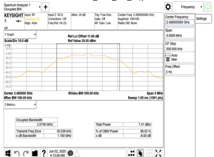
BLE 2M0BW 6dB_BLE_2M_HighCH39-2480
