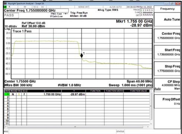
Band Edge_Band4_20MHz_QPSK_RB100_0_CH20300
