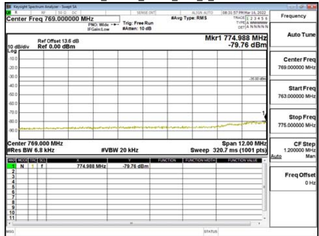
Band13_10MHz_QPSK_RB1_0_CH23230
