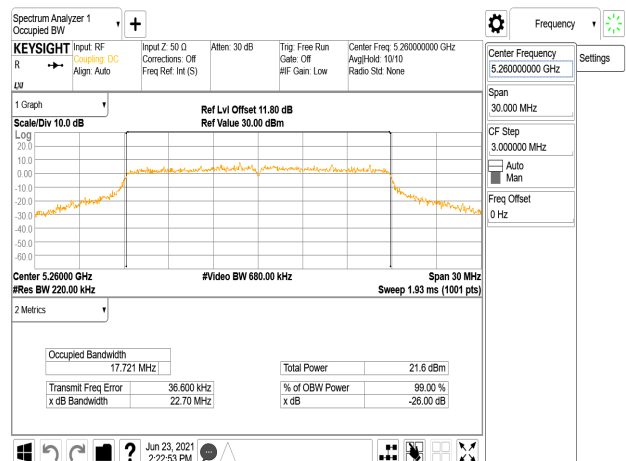
802.11n_20MHz_Chain1_5260MHz
