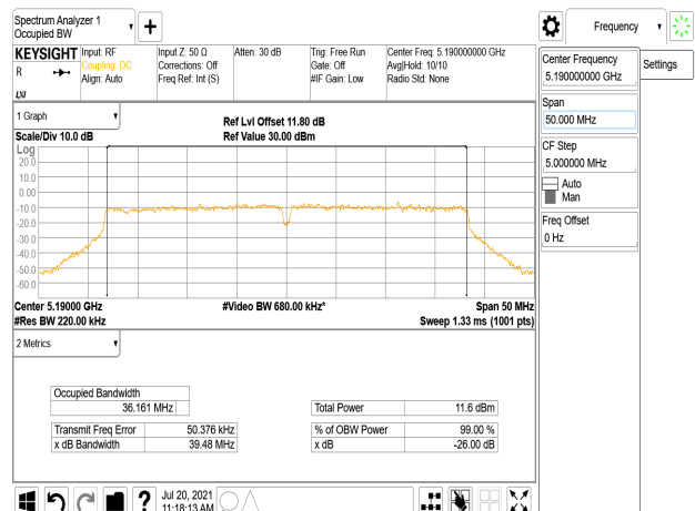
802.11n_40MHz_Test_Chain0
