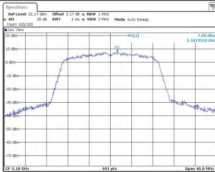
11N20BF_Ant1_5180
