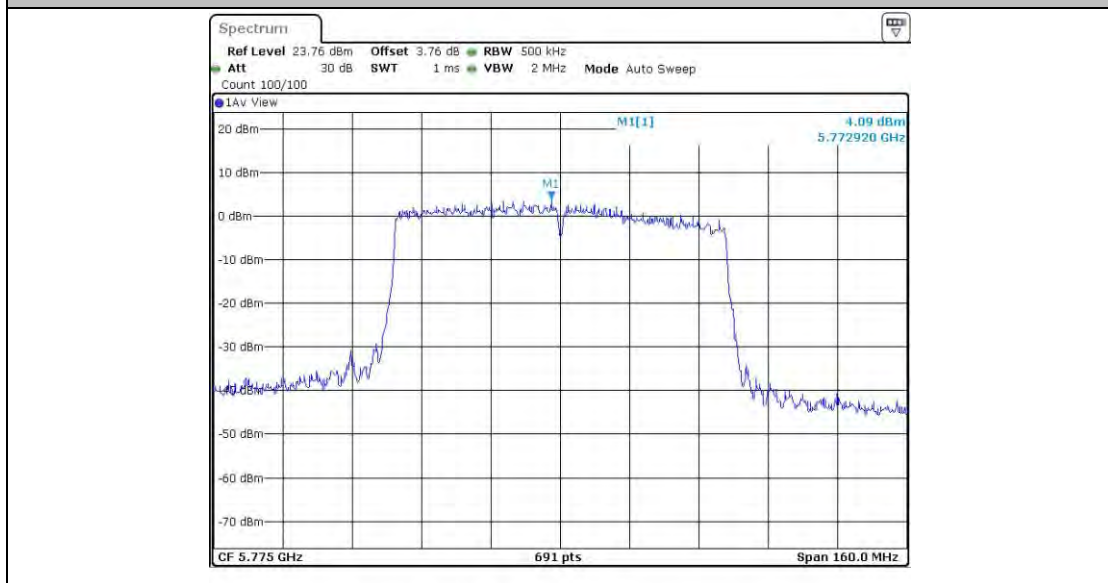
11AC80MIMO_Ant4_5775
