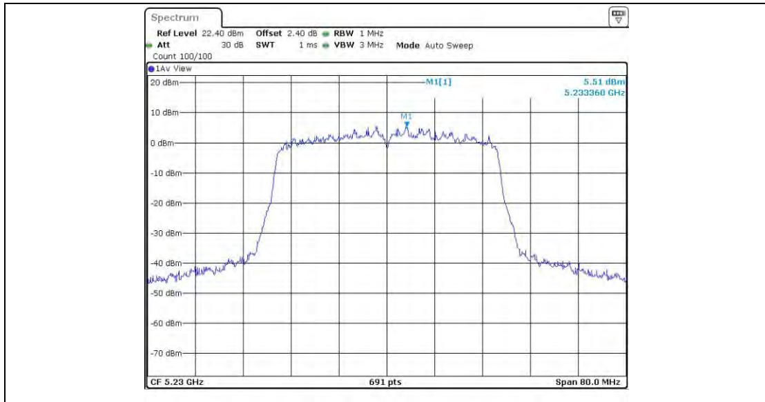
11N40BF_Ant3_5230
