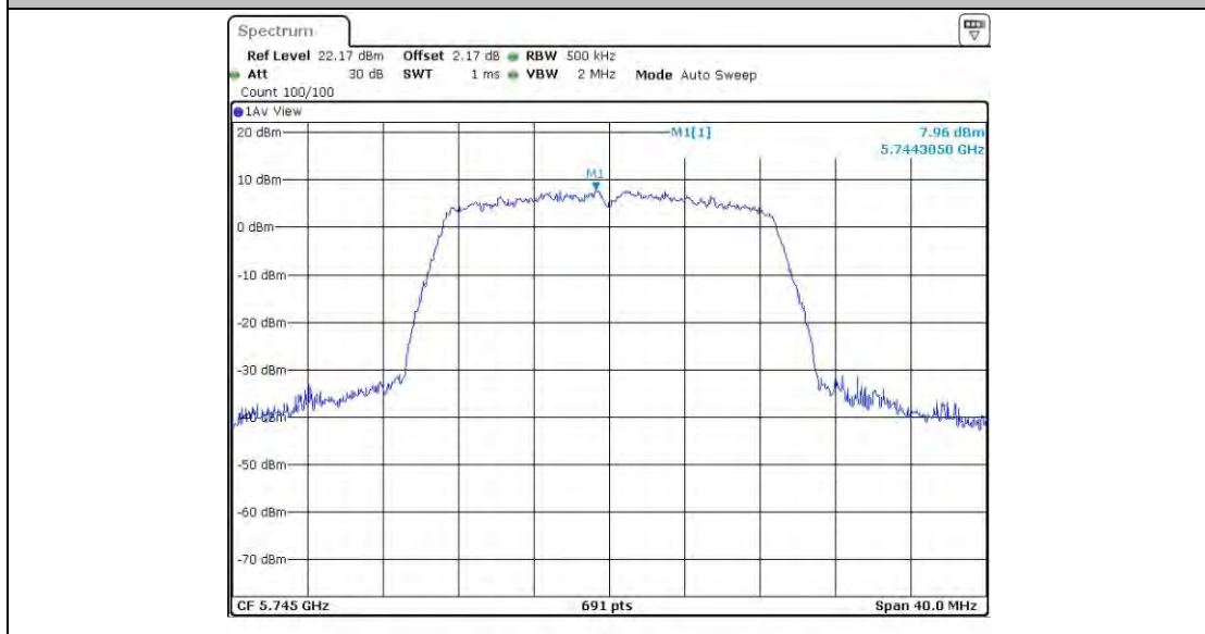
11N20MIMO_Ant4_5745
