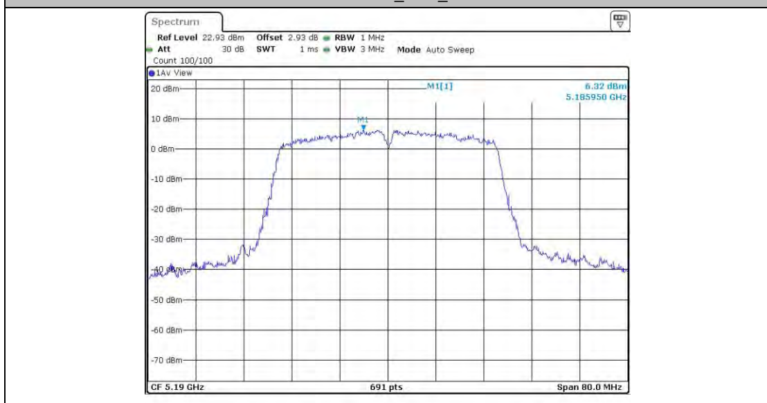
11AC40MIMO_Ant4_5190
