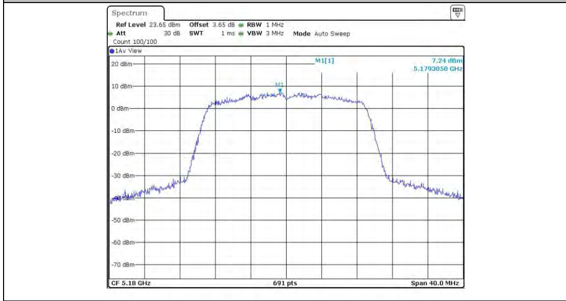
11AC20BF_Ant1_5180
