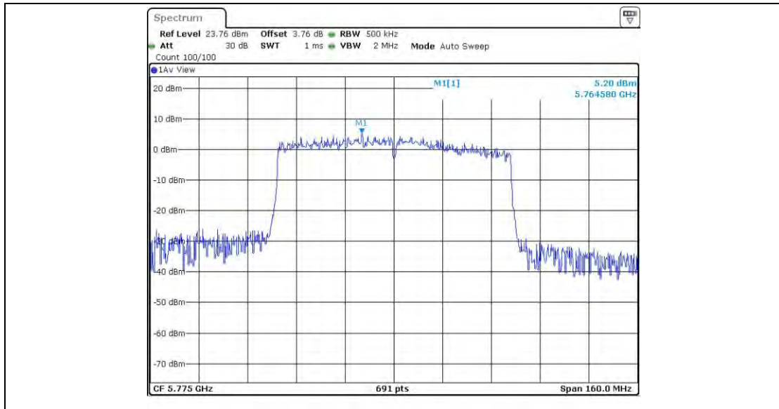
11AC80MIMO_Ant3_5775
