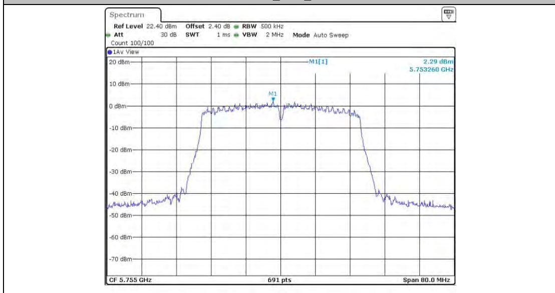
11N40BF_Ant1_5755
