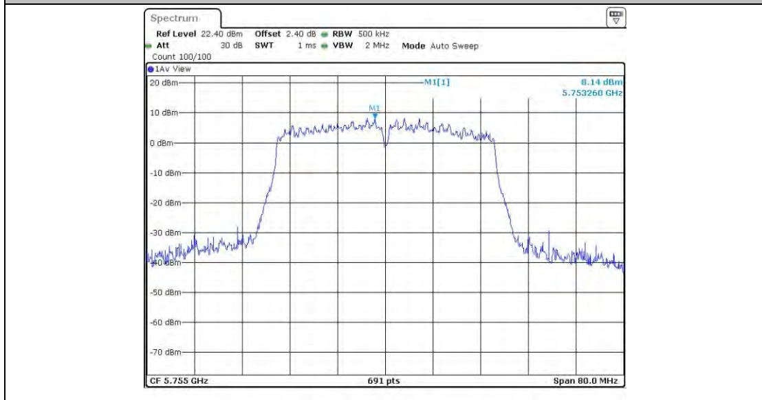
11N40MIMO_Ant3_5755
