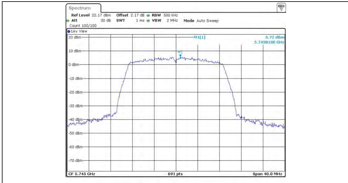
11N20BF_Ant1_5745
