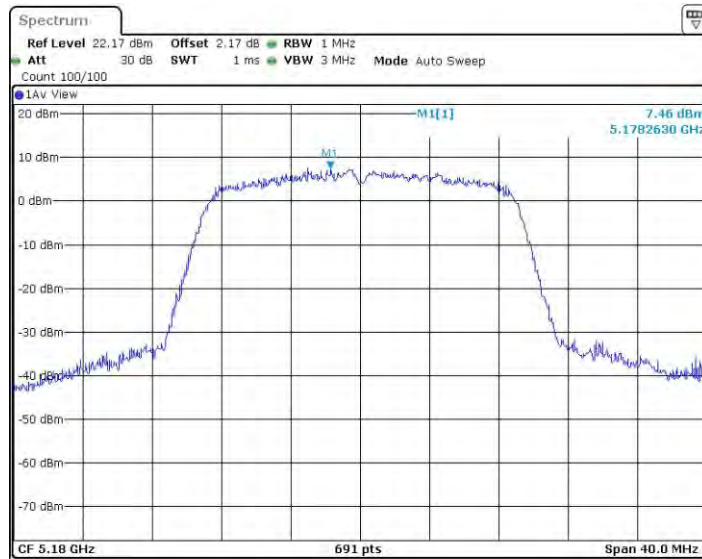
11N20BF_Ant2_5180
