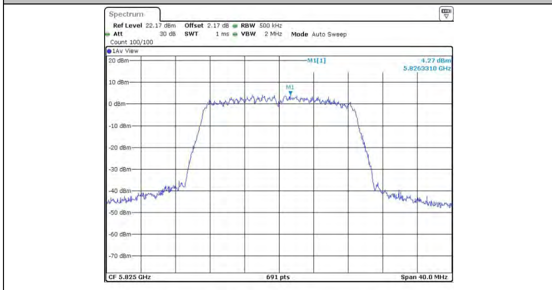
11N20BF_Ant3_5825
