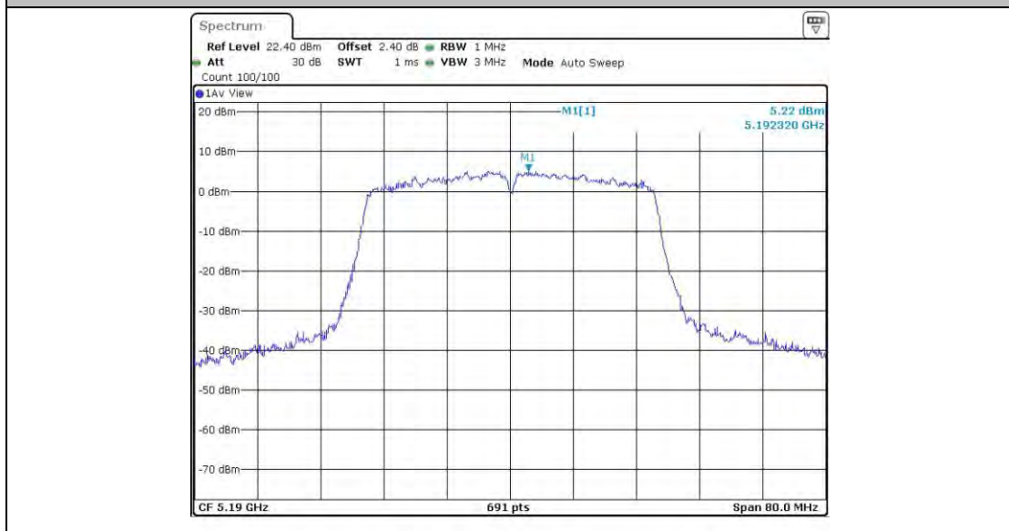
11N40MIMO_Ant4_5190
