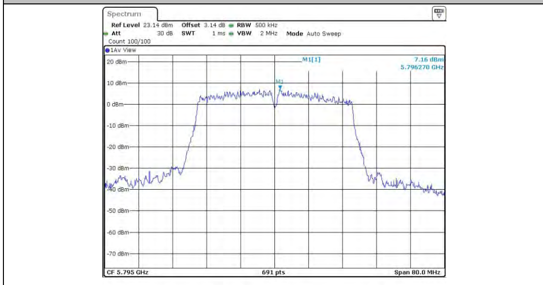
11AC40MIMO_Ant3_5795
