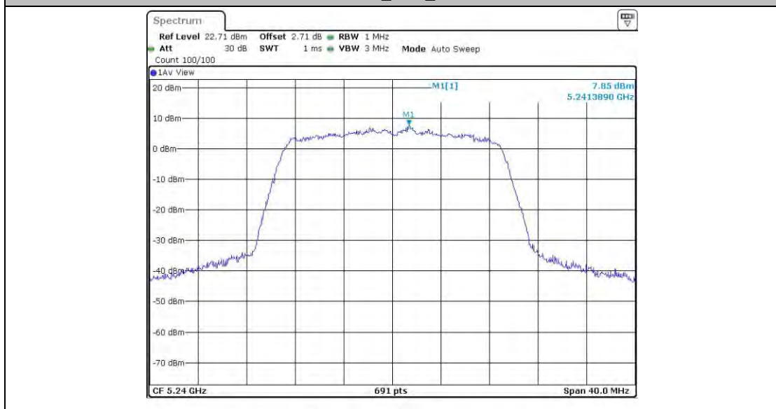
11N20BF_Ant1_5240
