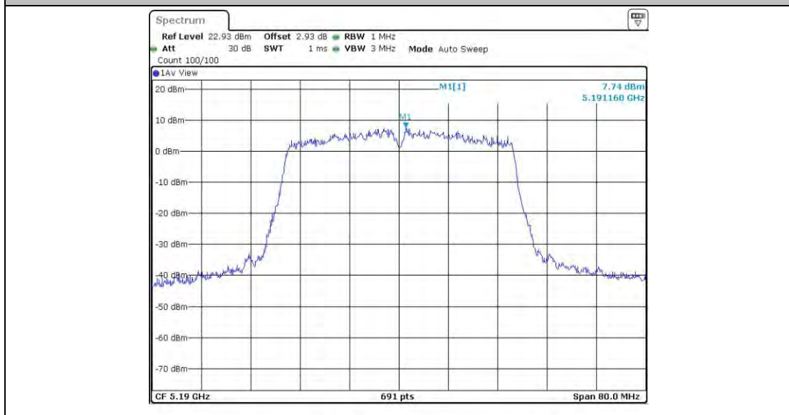
11AC40MIMO_Ant3_5190
