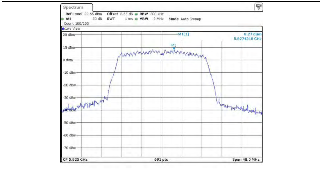
11AC20MIMO_Ant3_5825
