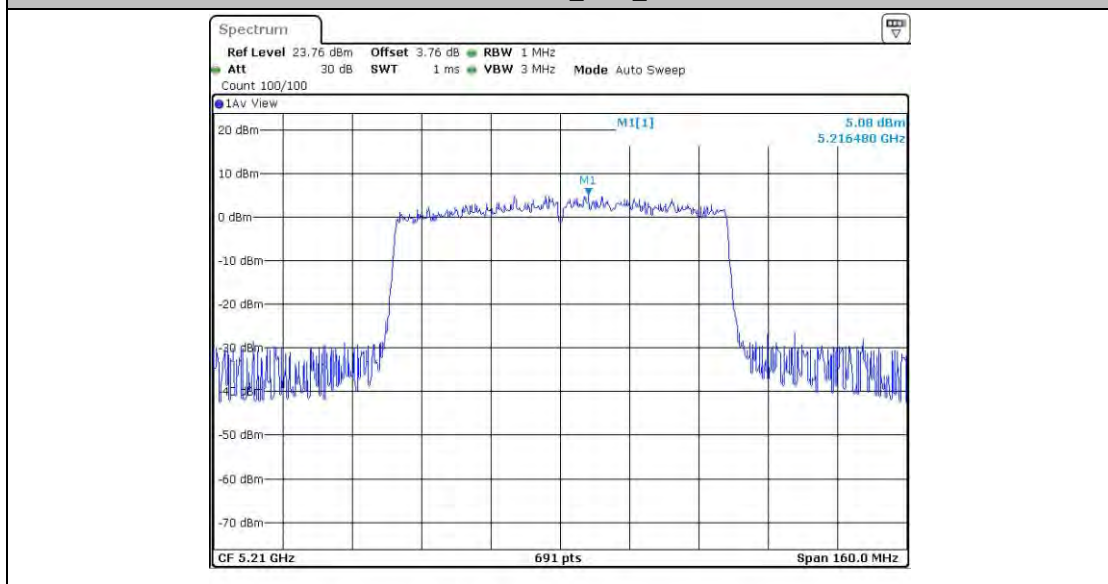
11AC80MIMO_Ant3_5210
