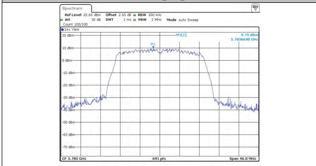
11AC20MIMO_Ant3_5785
