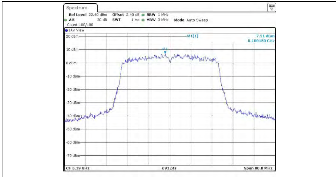
11N40MIMO_Ant3_5190
