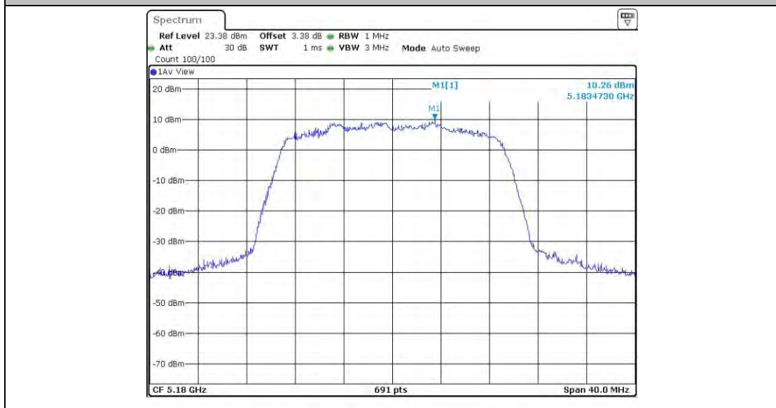
11AC20MIMO_Ant3_5180
