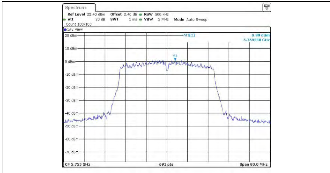
11N40BF_Ant2_5755
