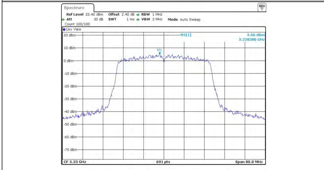
11N40BF_Ant2_5230
