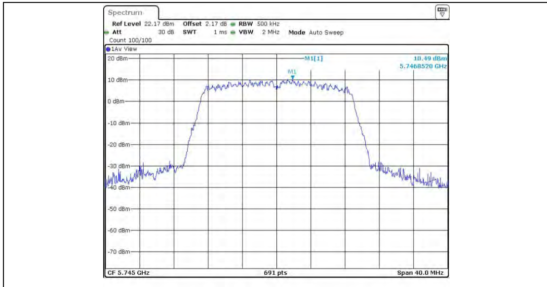
11N20MIMO_Ant3_5745
