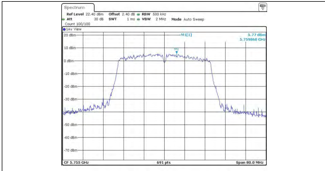
11N40MIMO_Ant4_5755
