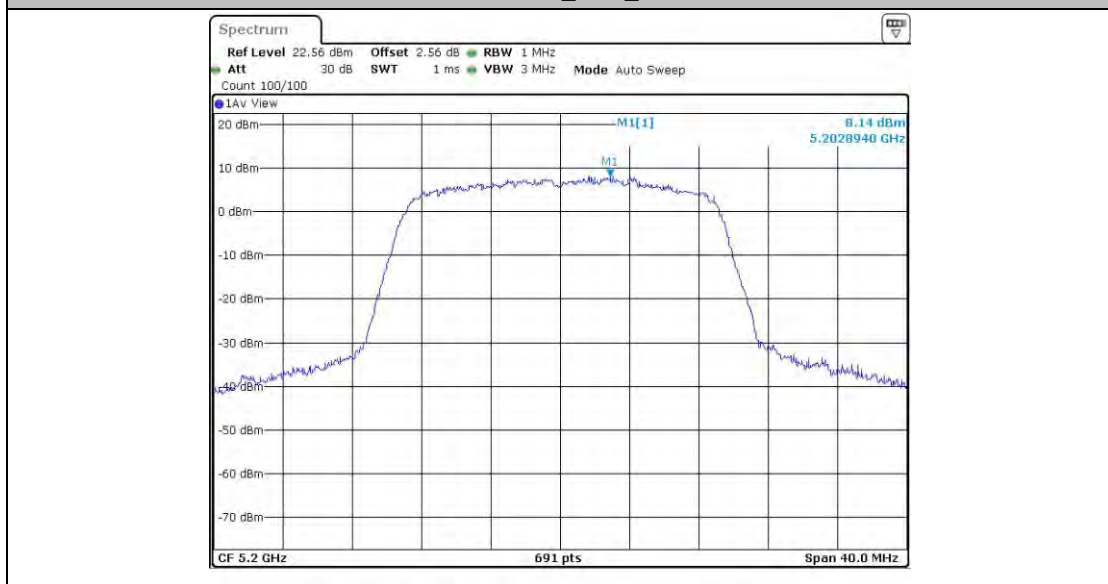
11N20MIMO_Ant4_5200
