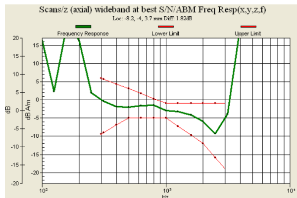
Fig. 9.14 WCDMA II Ch9400
