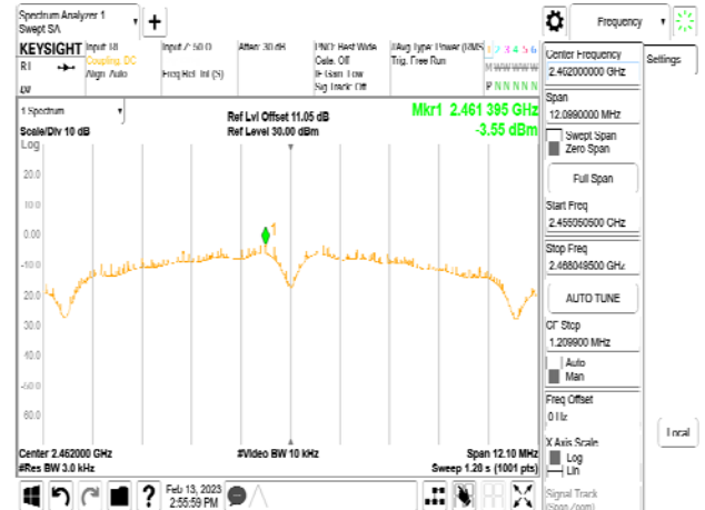
802.11b_20MHz_Chain1_2462MHz
