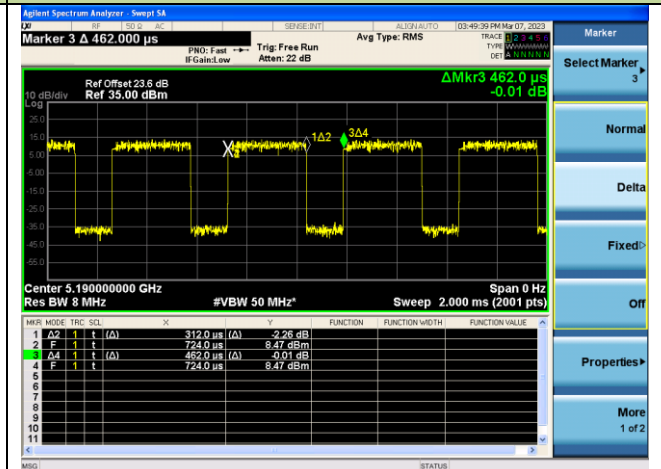
802.11ax-HE40 (T = 312.0us)
