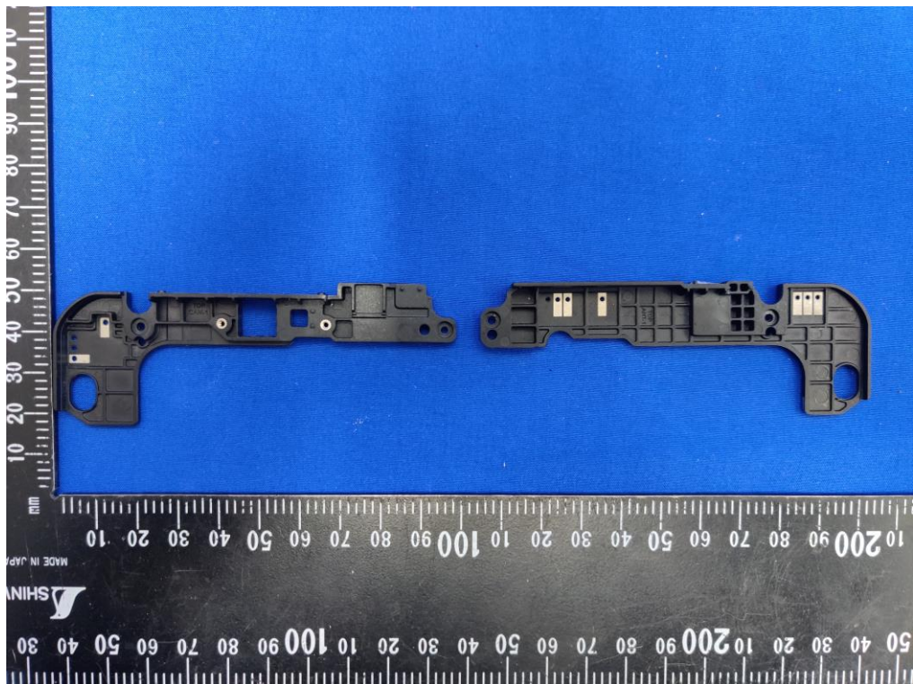
(30) EUT Photo
