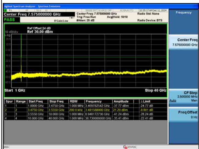
CSE_MIMO(ANT5)_n77(K)_30KHz_QPSK_70M CH634332_1RB@1_
