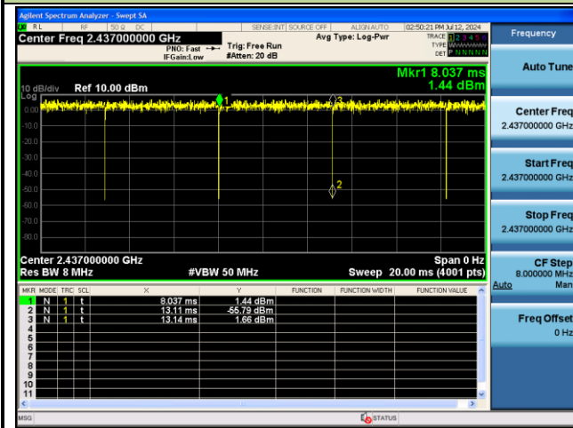
802.11ax-HE20_106 Tone_RU106
