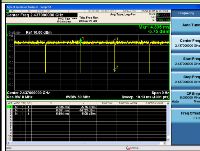
802.11ax-HE40_484 Tone_RU130
