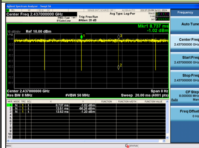
802.11ax-HE40_484 Tone_RU130
