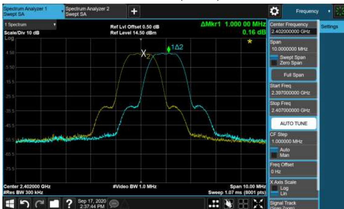
Mode 2 CH00(2402MHz)
