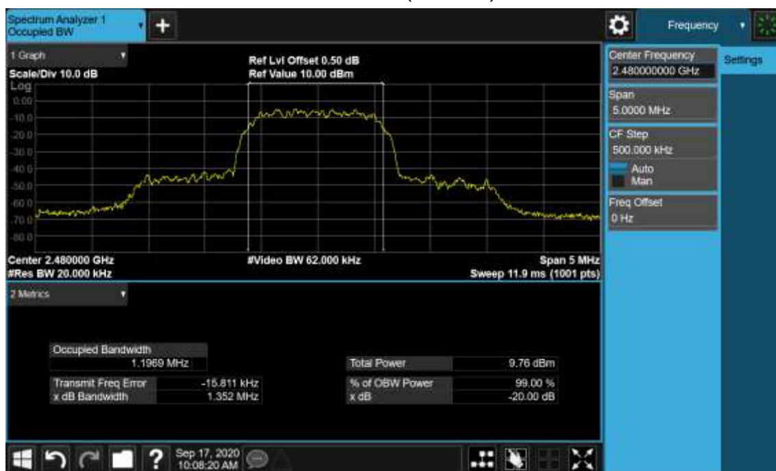
Mode 2 CH78(2480MHz)
