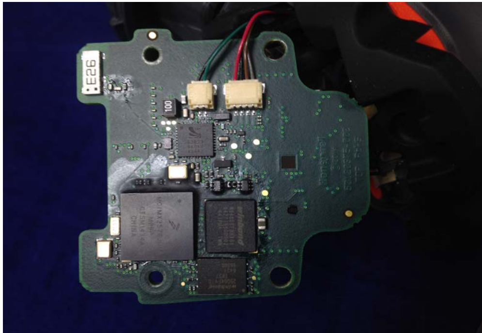
(4) EUT Photo
