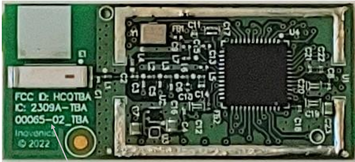
TBA Module - Topside
