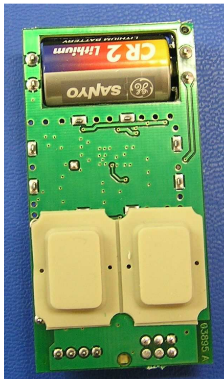
PCB bottomside
