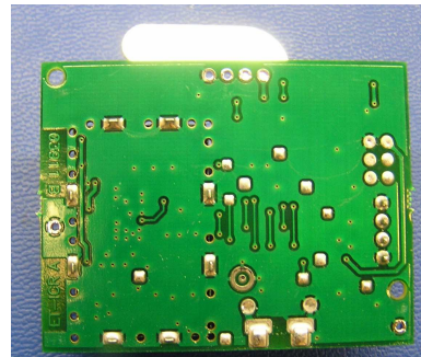
PCB bottomside
