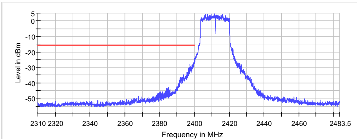
Band Edge
