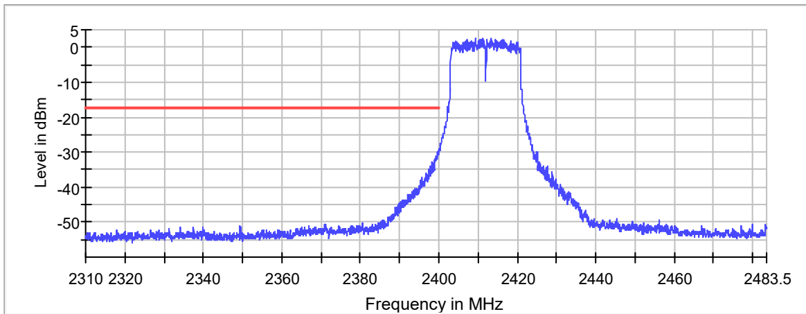
Band Edge
