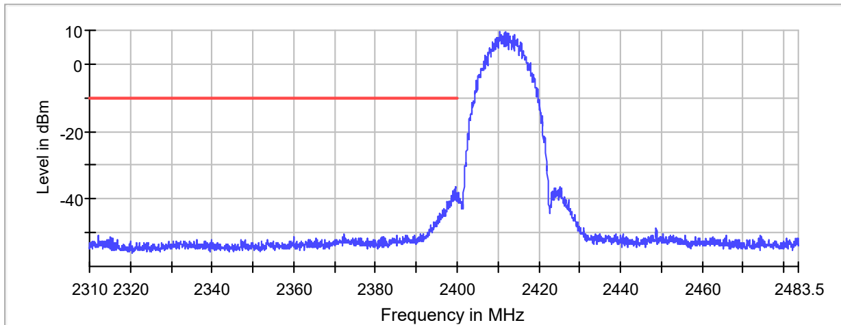
Band Edge
