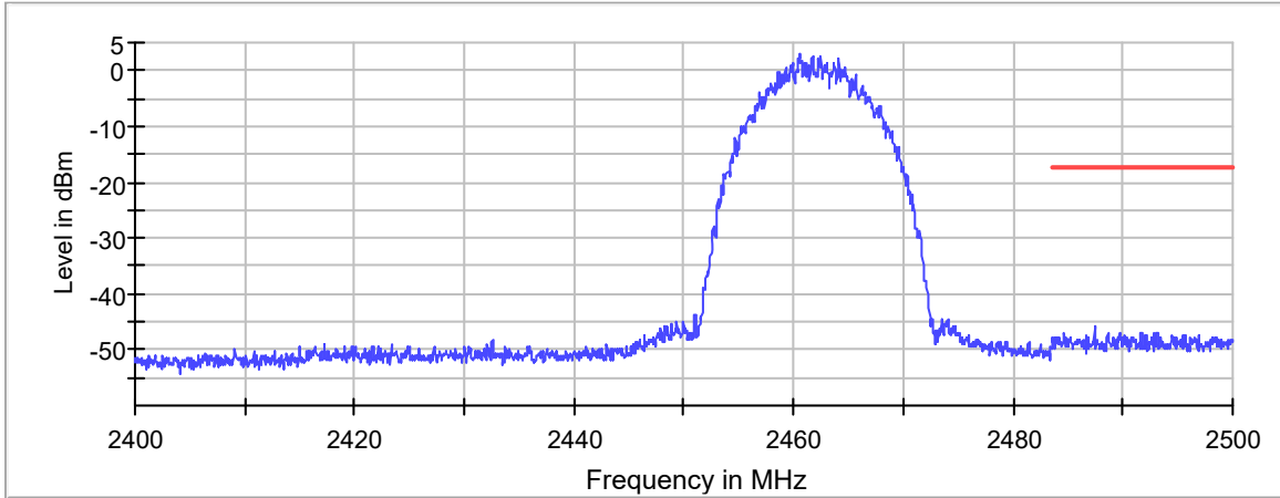
Band Edge
