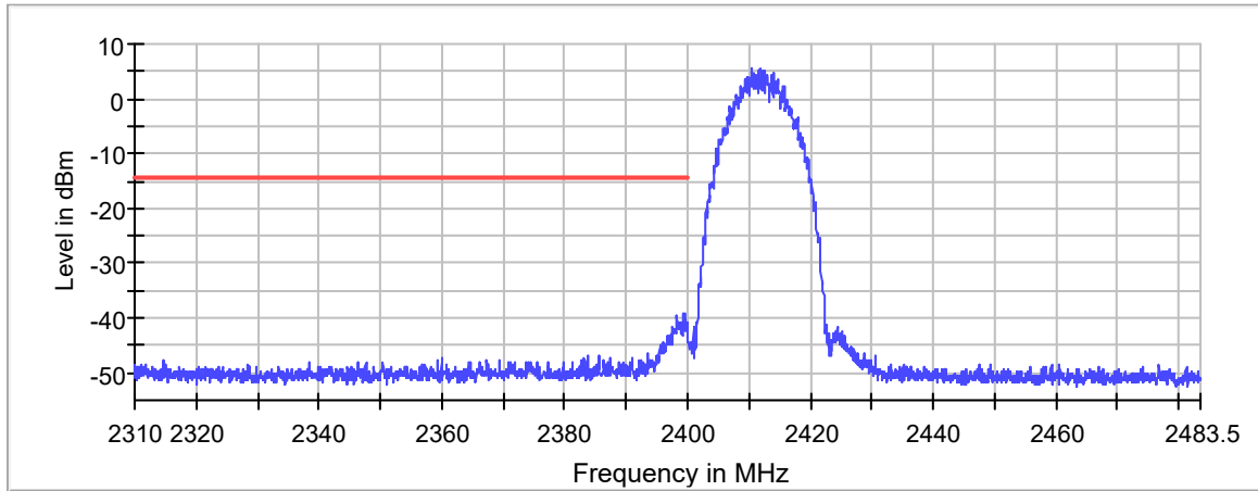
Band Edge
