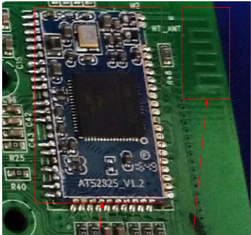
BT module
