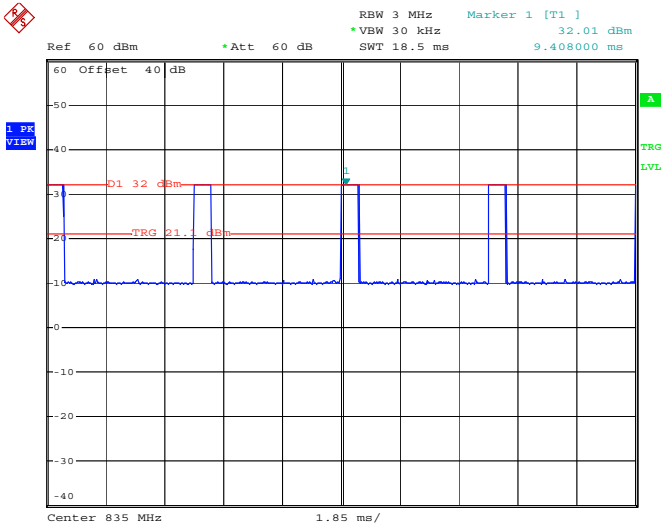
835MHz - GSM
