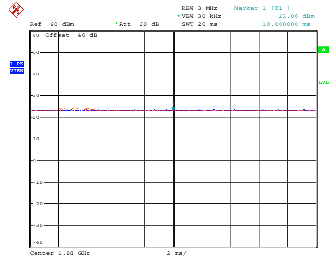
1880MHz - WCDMA
