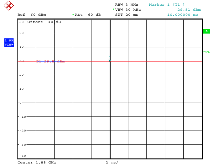
1880MHz - CW
