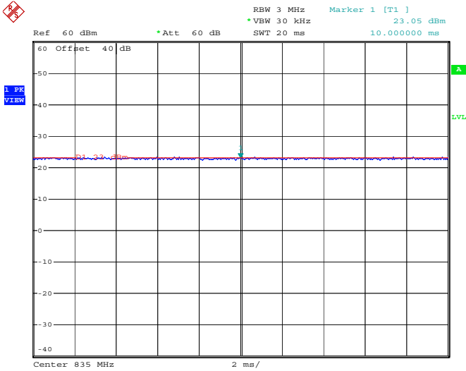
835MHz - WCDMA
