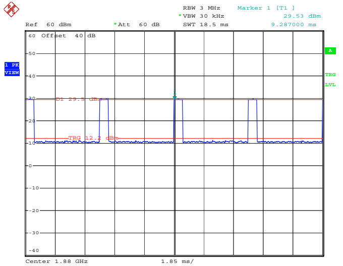
1880MHz - GSM
