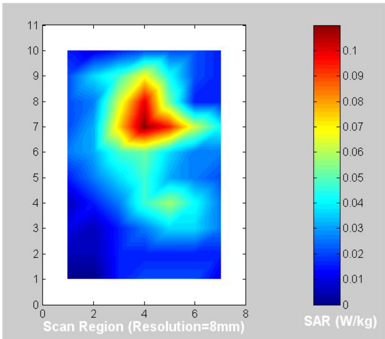
(d) 5.80 GHz turbo mode (see Table 10 for the peak 1-g SAR).
