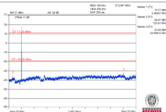
Chain 1 : CH 11
