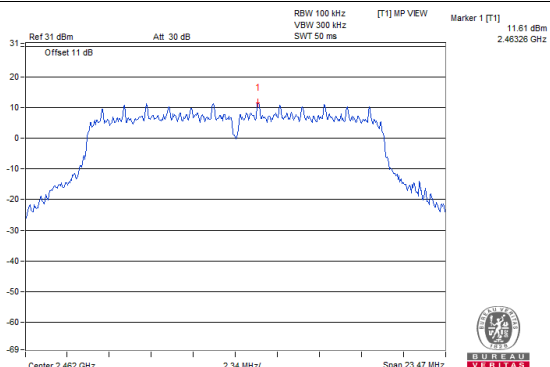
Chain 1 : CH 11
