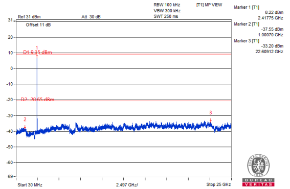
Chain 1 : CH 1
