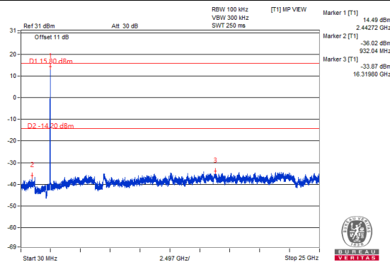
Chain 1 : CH 6
