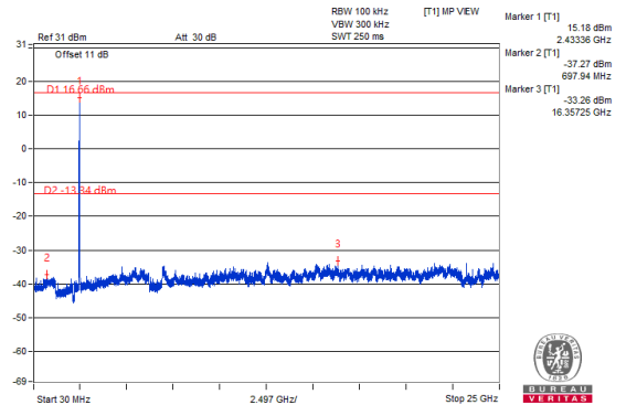
Chain 1 : CH 6
