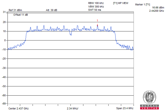
Chain 1 : CH 6
