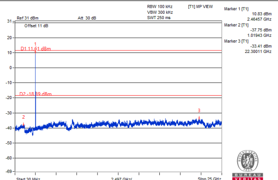
Chain 1 : CH 11
