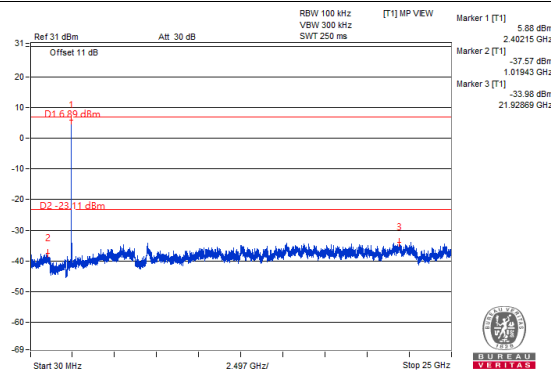
Chain 1 : CH 1
