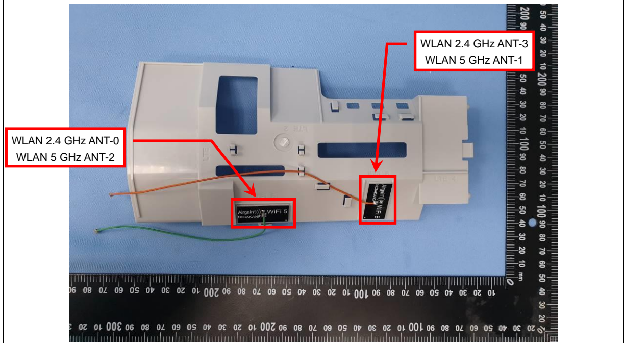
EUT Photo (4)
