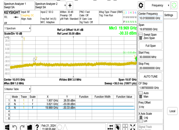
Band2_3MHz_QPSK_RB1_0_CH19185
