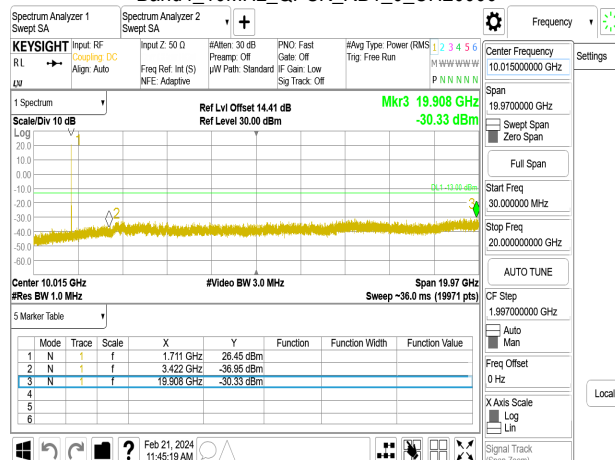
Band4_10MHz_QPSK_RB1_0_CH20175
