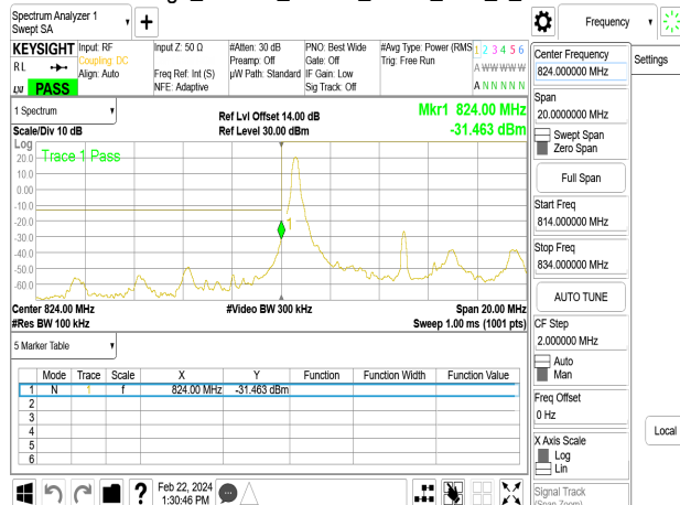
Band Edge_Band26_10MHz_QPSK_RB1_49_CH26990
