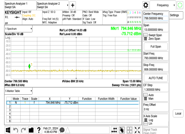
Band13_10MHz_QPSK_RB50_0_CH23230
