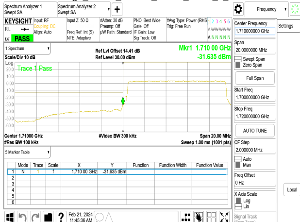
Band Edge_Band4_10MHz_QPSK_RB50_0_CH20000
