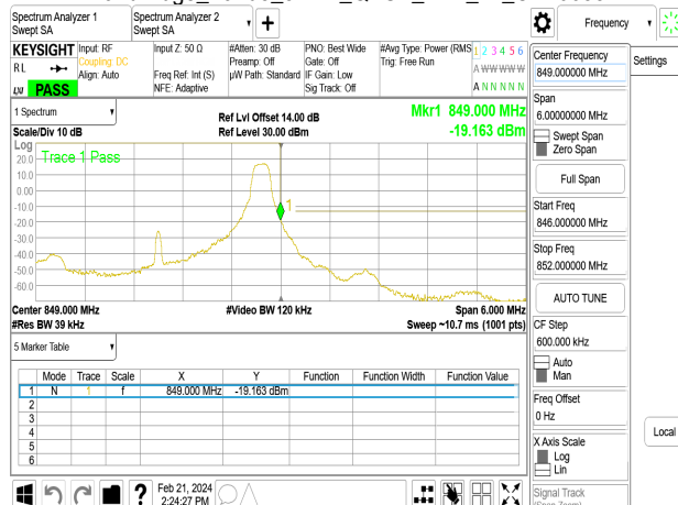
Band Edge_Band5_3MHz_QPSK_RB1_14_CH20635
