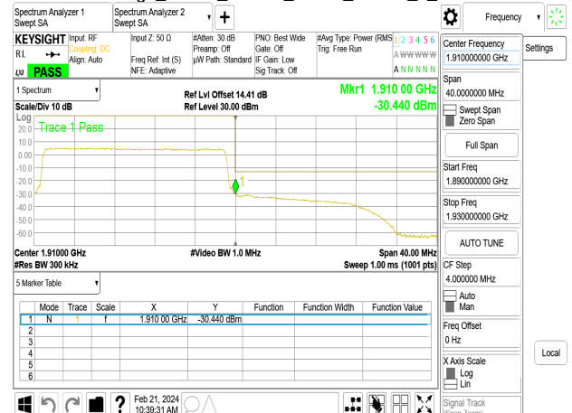
Band Edge_Band2_20MHz_QPSK_RB100_0_CH19100
