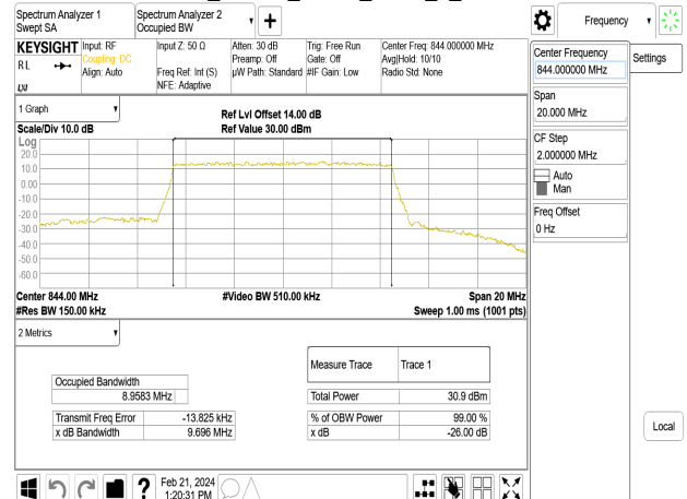
Band5_10MHz_QPSK_RB50_0_CH20600
