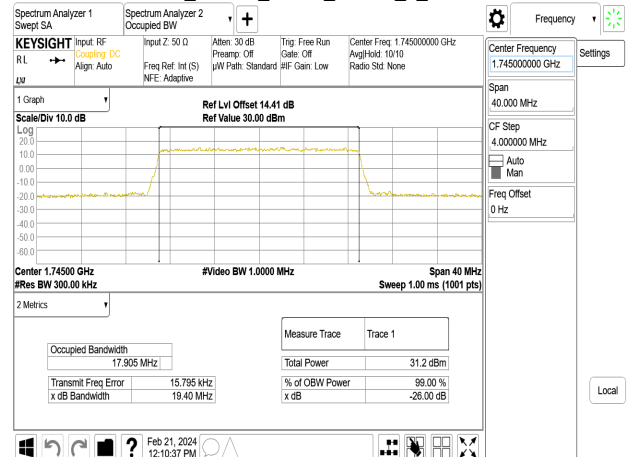
Band4_20MHz_QPSK_RB100_0_CH20300
