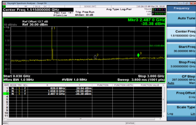
30MHz~3GHz_Band5_10MHz_QPSK_1_0_LowCH2045 0-829
