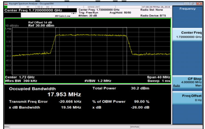
Band4 20MHz 16QAM 100 0 LowCH20050-1720
