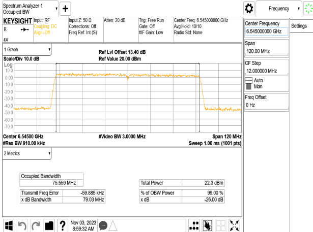
802.11ac_80MHz_Chain2_6545MHz
