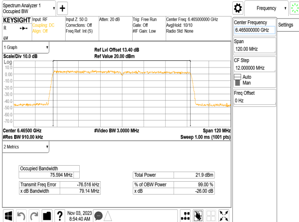
802.11ac_80MHz_Chain1_6465MHz
