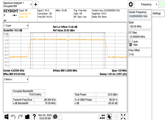
802.11ac_80MHz_Chain0_6625MHz
