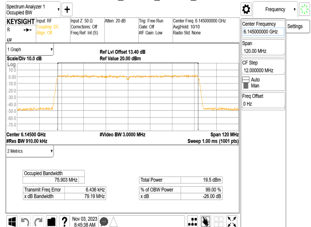
802.11ac_80MHz_Chain2_6145MHz
