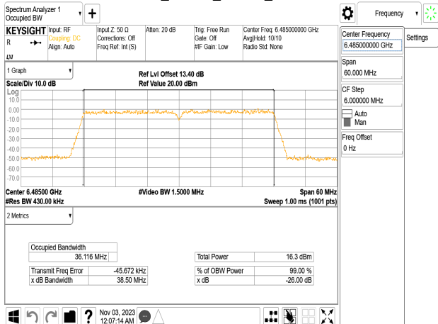
802.11n_40MHz_Chain2_6485MHz
