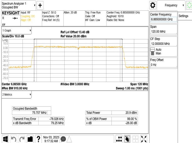
802.11ac_80MHz_Chain0_6865MHz
