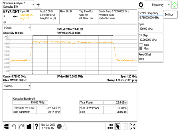
802.11ac_80MHz_Chain2_6785MHz
