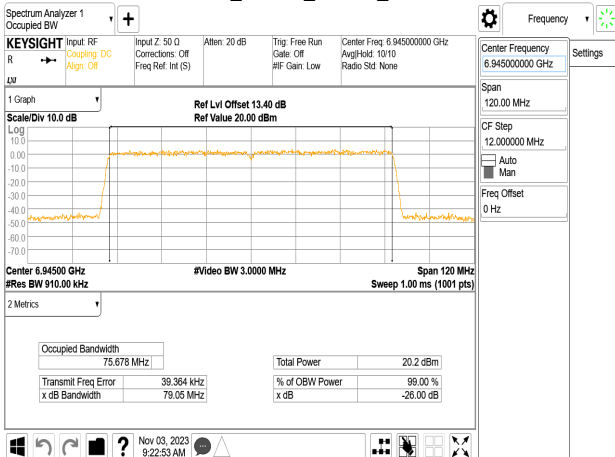
802.11ac_80MHz_Chain1_6945MHz
