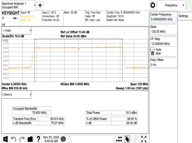
802.11ac_80MHz_Chain0_6385MHz
