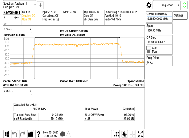
802.11ac_80MHz_Chain1_5985MHz
