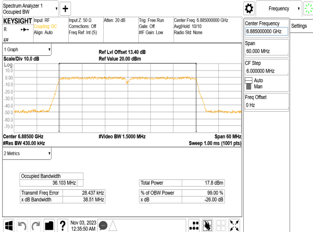
802.11n_40MHz_Chain3_6885MHz
