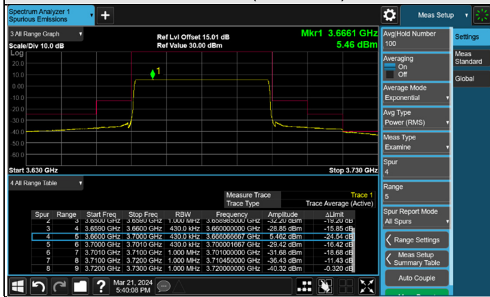
CH 645332 (3679.98 MHz)
