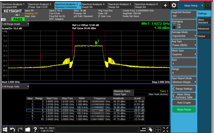
CH 641666 (3624.99 MHz)
