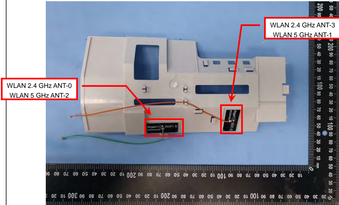
EUT Photo (4)
