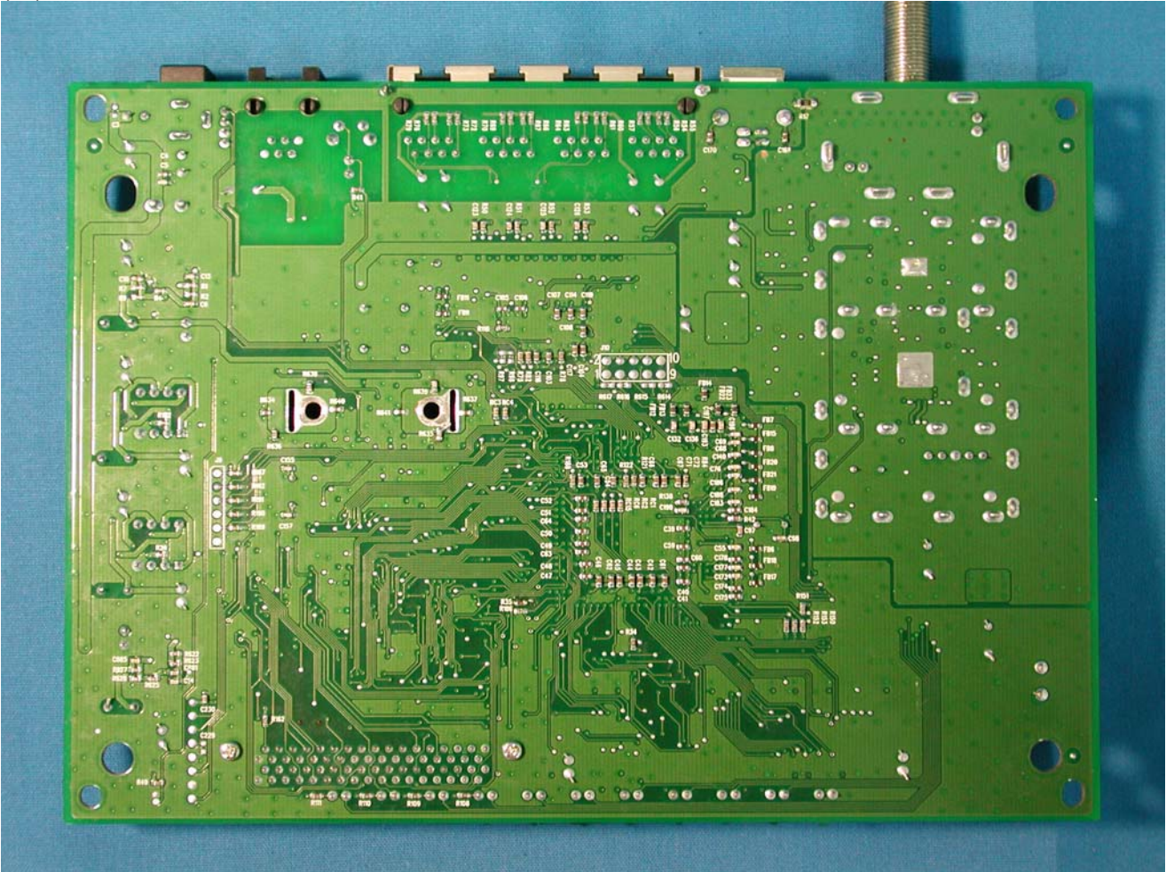
(14) EUT Photo
