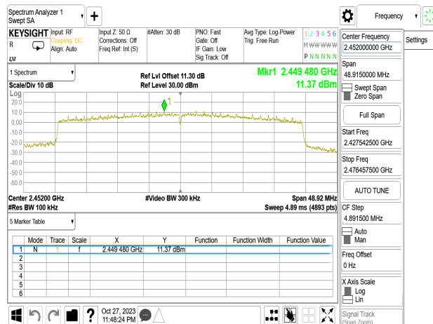
802.11be_40MHz_Chain3_2452MHz
