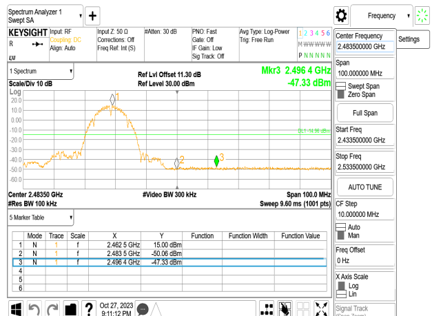
802.11b_20MHz_Chain2_2462MHz
