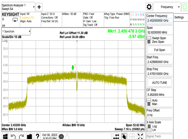
802.11be_40MHz_Chain0_2452MHz
