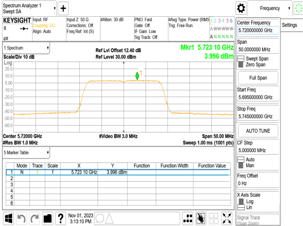
802.11a_20MHz_Chain2_5720MHz_UNII 3
