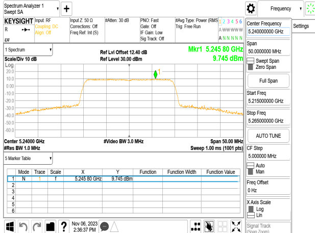
802.11be_20MHz_Chain3_5240MHz
