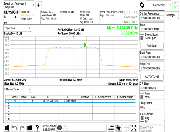
802.11be_20MHz_Chain3_5720MHz_UNII 3
