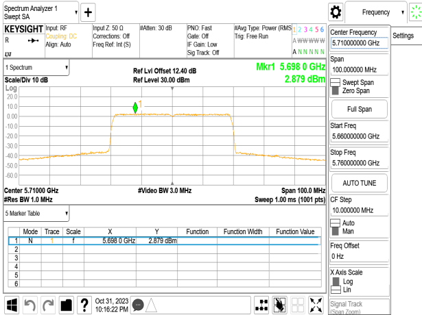
802.11be_40MHz_Chain3_5710MHz_UNII 3
