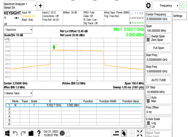
802.11be_40MHz_Chain2_5550MHz
