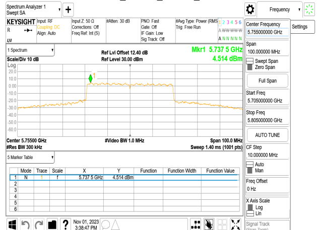
802.11be_40MHz_Chain0_5755MHz
