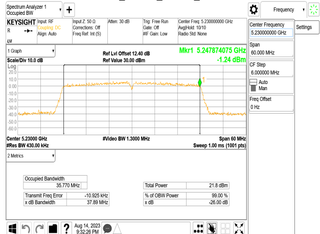
802.11n_40MHz_Chain2_5230MHz
