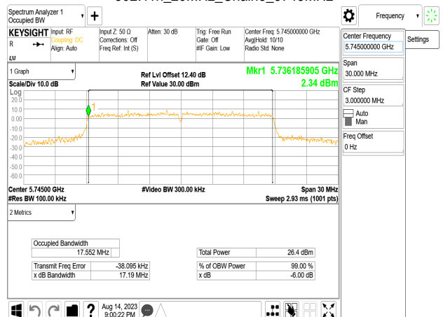
802.11n_20MHz_Chain3_5745MHz
