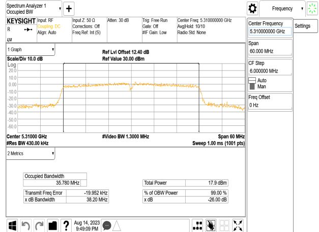
802.11n_40MHz_Chain3_5310MHz
