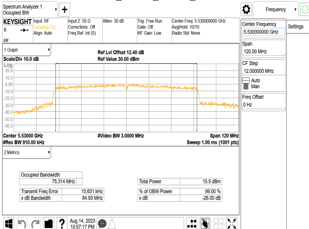
802.11ac_80MHz_Chain3_5530MHz
