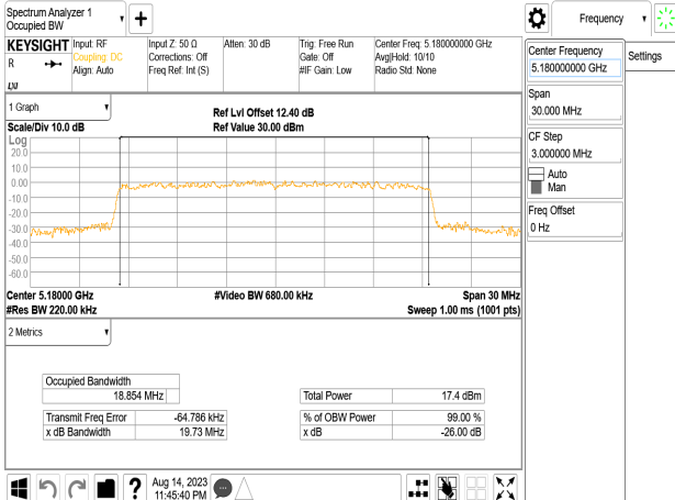
802.11be_20MHz_Chain0_5180MHz
