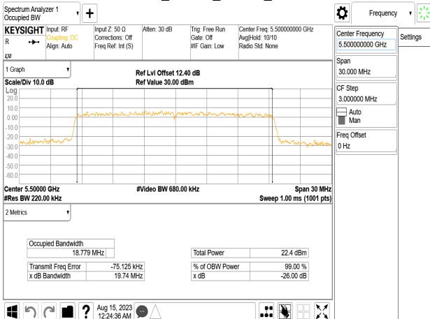
802.11be_20MHz_Chain0_5500MHz
