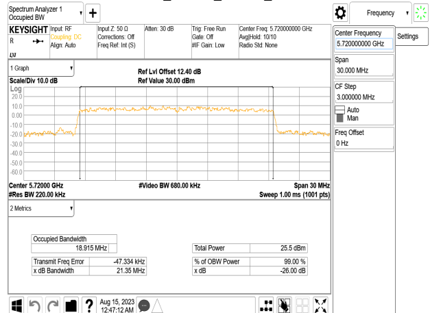
802.11be_20MHz_Chain0_5720MHz
