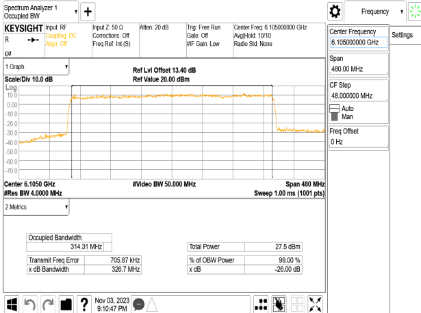
802.11be_320MHz_Chain0_6105MHz
