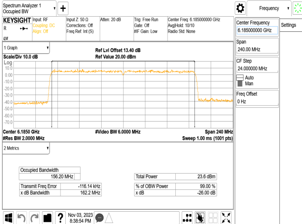
802.11be_160MHz_Chain3_6185MHz
