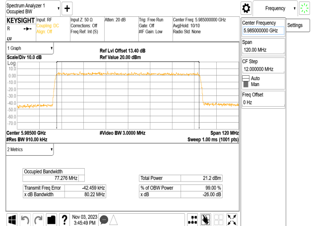
802.11be_80MHz_Chain3_5985MHz
