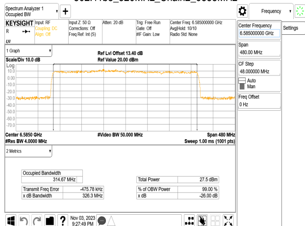
802.11be_320MHz_Chain2_6585MHz
