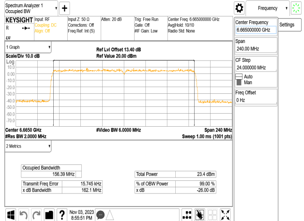
802.11be_160MHz_Chain3_6665MHz
