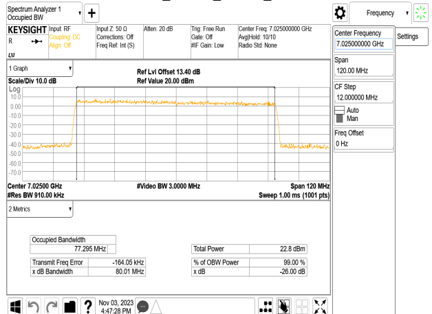
802.11be_80MHz_Chain1_7025MHz
