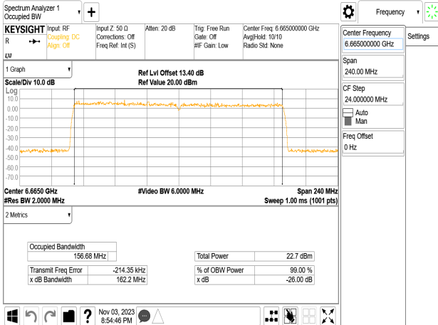
802.11be_160MHz_Chain0_6665MHz
