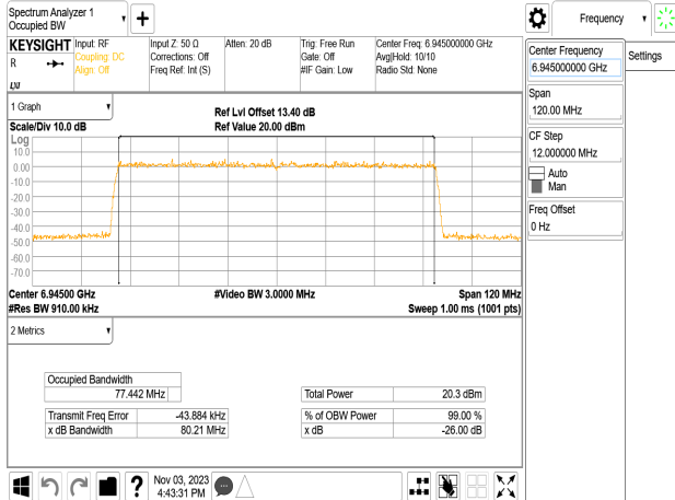
802.11be_80MHz_Chain3_6945MHz
