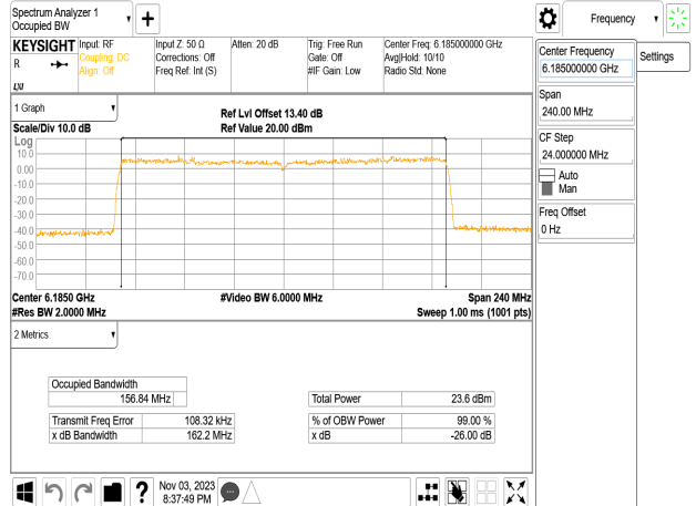
802.11be_160MHz_Chain0_6185MHz
