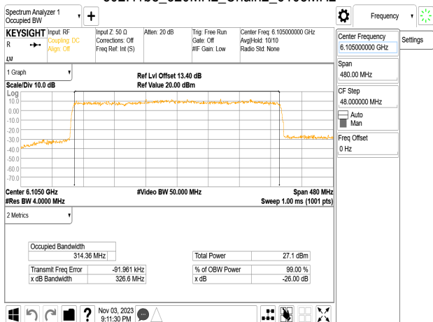
802.11be_320MHz_Chain2_6105MHz
