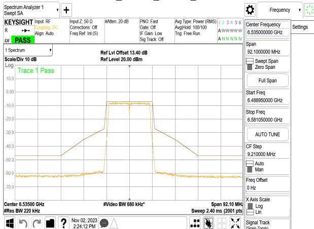
802.11a_20MHz_Chain2_6535MHz
