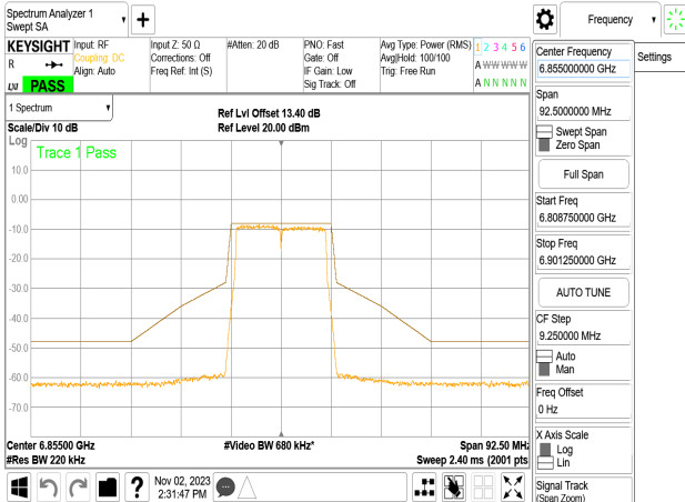
802.11a_20MHz_Chain0_6855MHz
