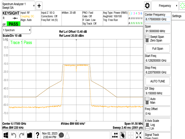
802.11a_20MHz_Chain1_6175MHz
