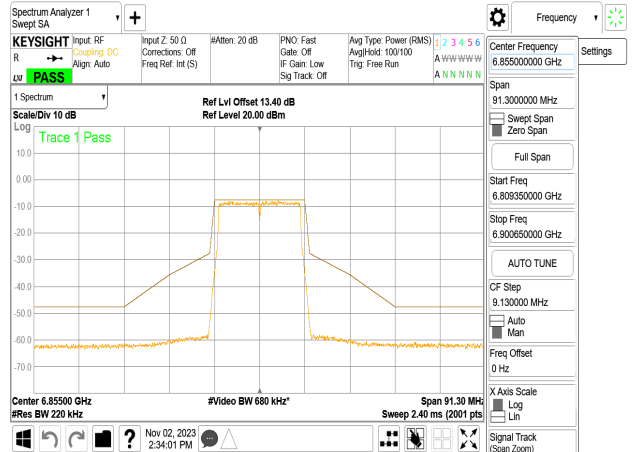
802.11a_20MHz_Chain3_6855MHz
