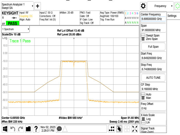
802.11a_20MHz_Chain1_6695MHz
