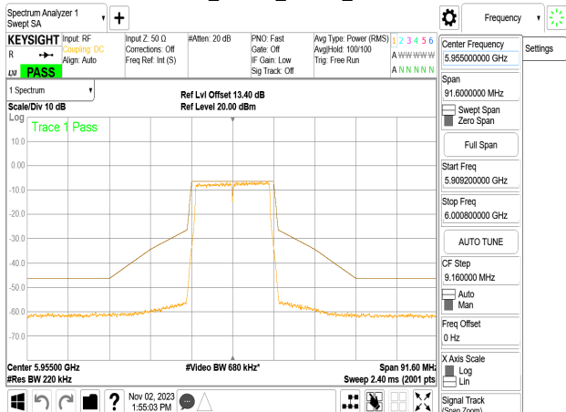
802.11a_20MHz_Chain2_5955MHz
