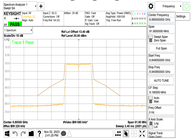
802.11a_20MHz_Chain1_6895MHz
