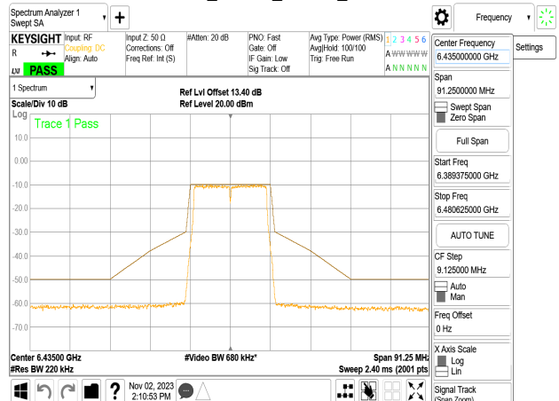
802.11a_20MHz_Chain2_6435MHz
