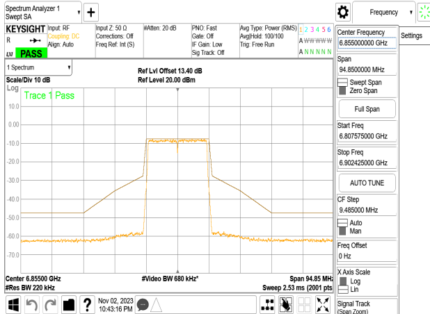
802.11n_20MHz_Chain2_6855MHz
