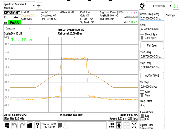
802.11n_20MHz_Chain1_6535MHz
