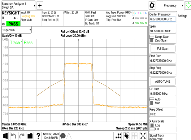
802.11n_20MHz_Chain1_6875MHz
