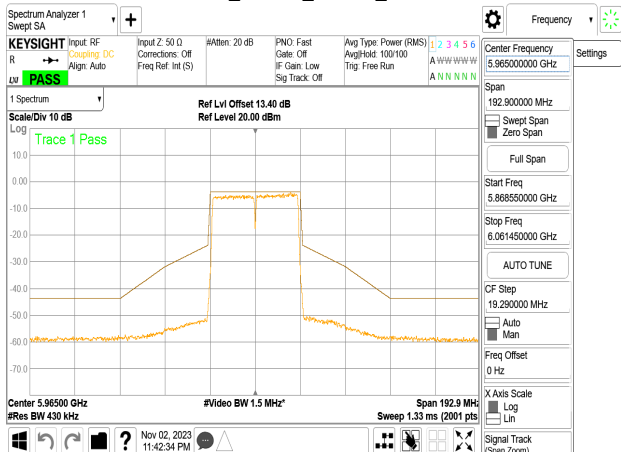
802.11n_40MHz_Chain0_5965MHz
