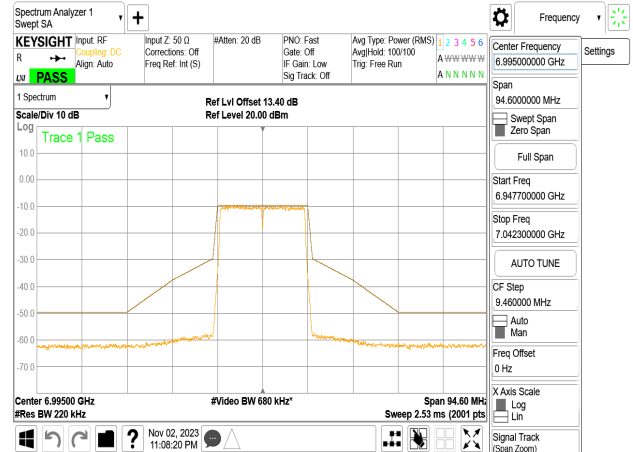
802.11n_20MHz_Chain2_6995MHz
