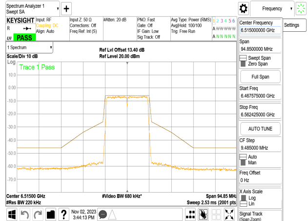
802.11n_20MHz_Chain2_6515MHz
