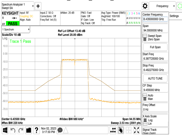
802.11n_20MHz_Chain1_6435MHz
