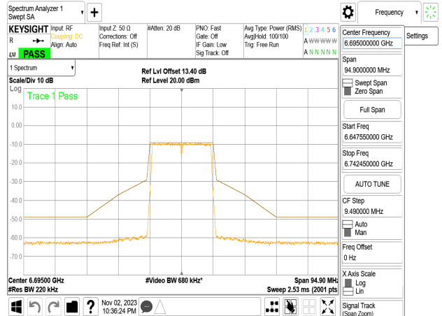
802.11n_20MHz_Chain0_6695MHz
