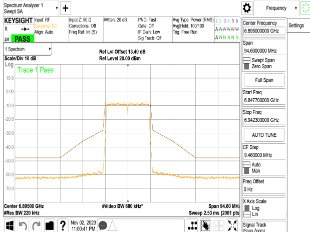
802.11n_20MHz_Chain0_6895MHz
