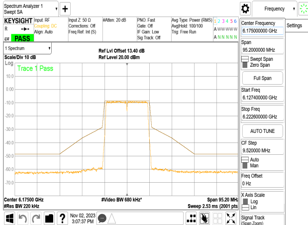
802.11n_20MHz_Chain3_6175MHz
