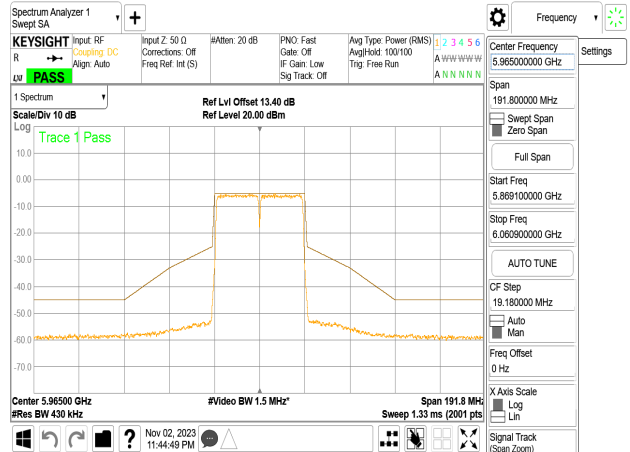
802.11n_40MHz_Chain3_5965MHz
