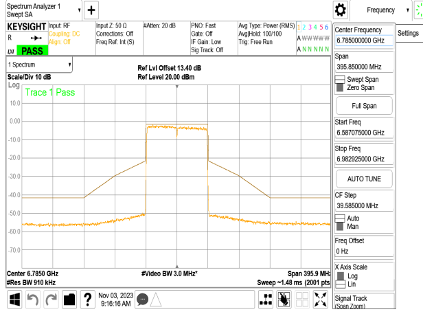
802.11ac_80MHz_Chain2_6785MHz
