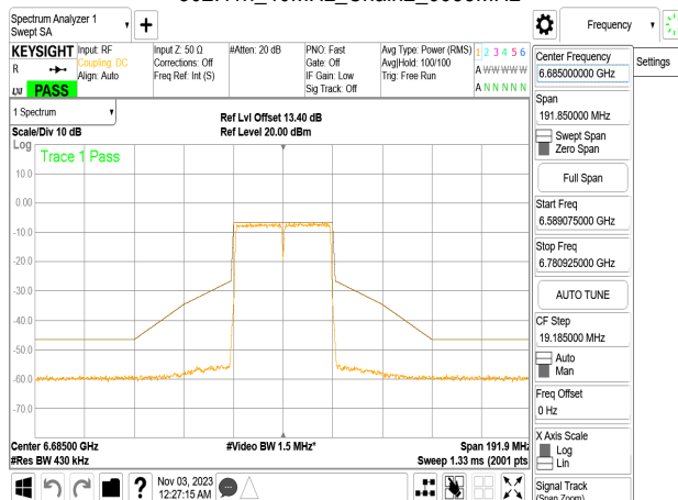
802.11n_40MHz_Chain2_6685MHz
