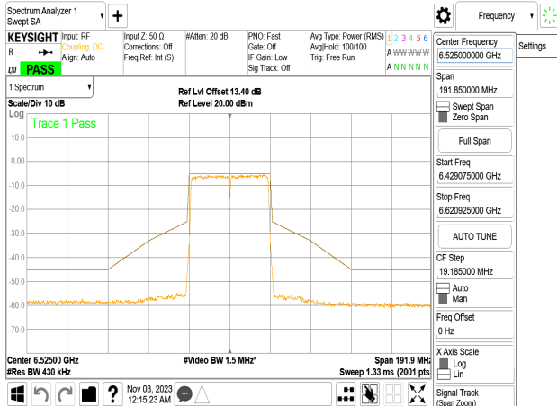
802.11n_40MHz_Chain1_6525MHz
