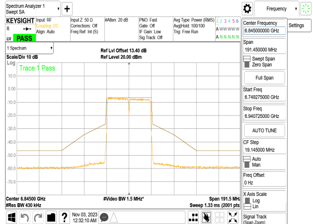
802.11n_40MHz_Chain1_6845MHz
