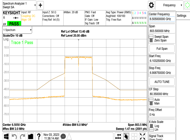
802.11ac_160MHz_Chain3_6505MHz
