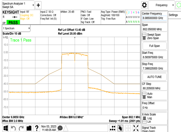
802.11ac_160MHz_Chain0_6985MHz
