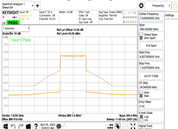
802.11ac_80MHz_Chain2_7025MHz
