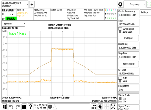
802.11be_40MHz_Chain2_6405MHz
