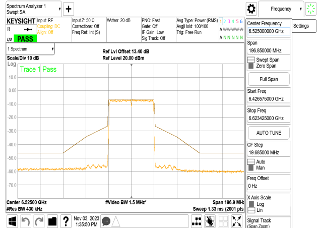
802.11be_40MHz_Chain2_6525MHz
