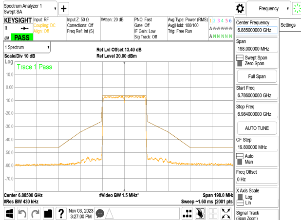
802.11be_40MHz_Chain1_6885MHz
