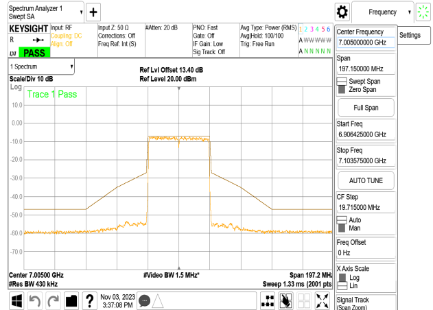
802.11be_40MHz_Chain2_7005MHz
