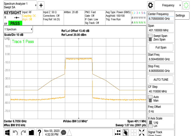
802.11be_80MHz_Chain3_6705MHz
