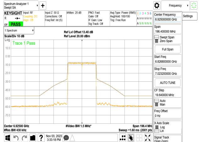
802.11be_40MHz_Chain3_6925MHz
