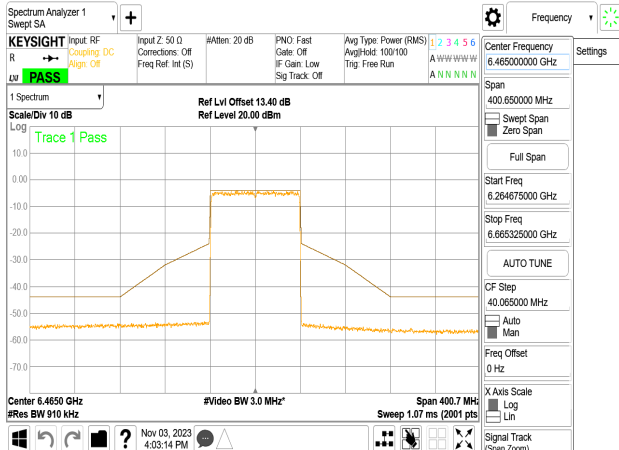
802.11be_80MHz_Chain3_6465MHz
