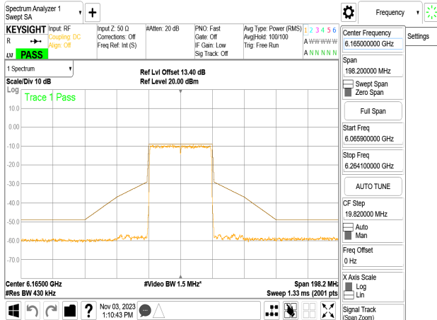
802.11be_40MHz_Chain3_6165MHz
