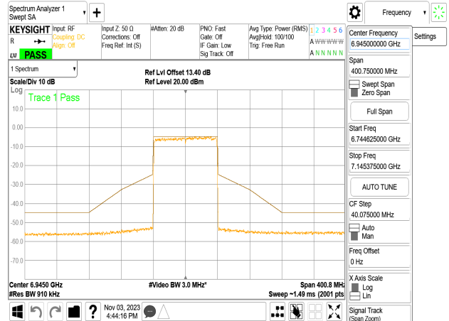
802.11be_80MHz_Chain0_6945MHz
