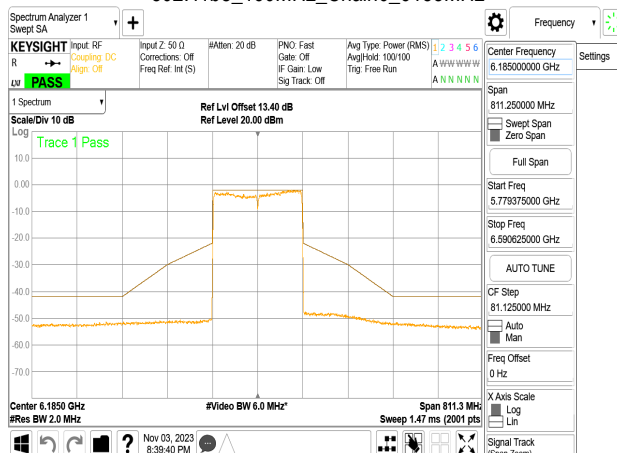
802.11be_160MHz_Chain0_6185MHz
