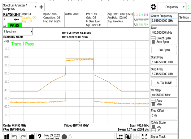
802.11be_80MHz_Chain1_6545MHz
