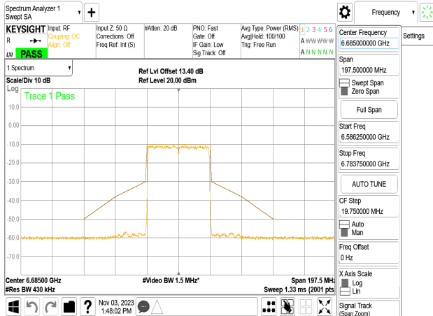
802.11be_40MHz_Chain3_6685MHz
