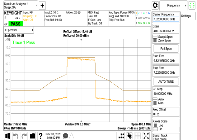
802.11be_80MHz_Chain1_7025MHz
